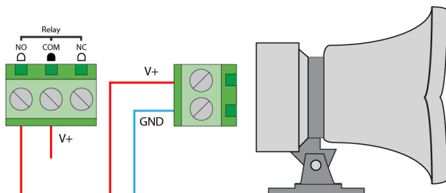
Схема подключения сирены к Relay V+ - напряжение питания, GND - земля
