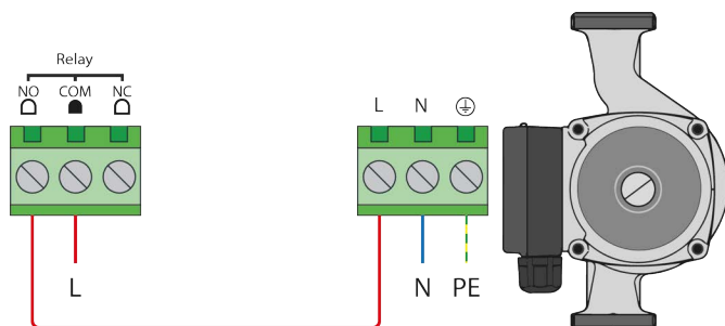
Схема подключения циркуляционного насоса к Relay L - напряжение питания (фаза), N - ноль, PE - заземление
