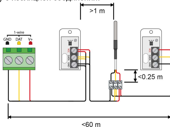
Схема подключения проводного датчика температуры MyHeat и датчика температуры в колбе MyHeat к шине 1-Wire.
