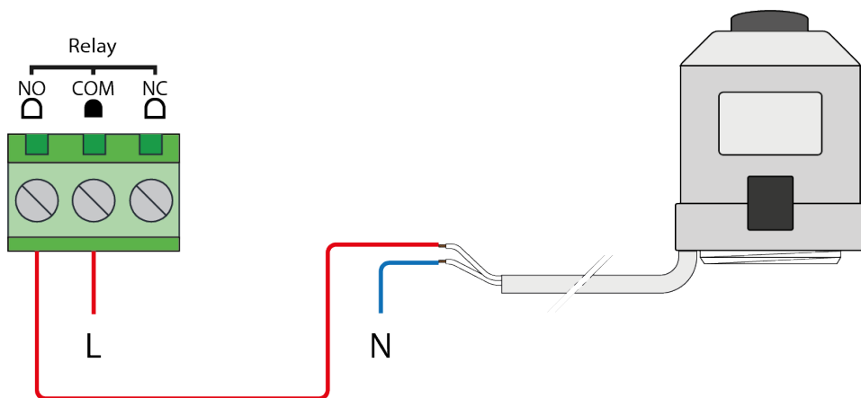
Схема подключения сервопривода электротермического двухпозиционного к Relay L - напряжение питания (фаза), N - ноль
